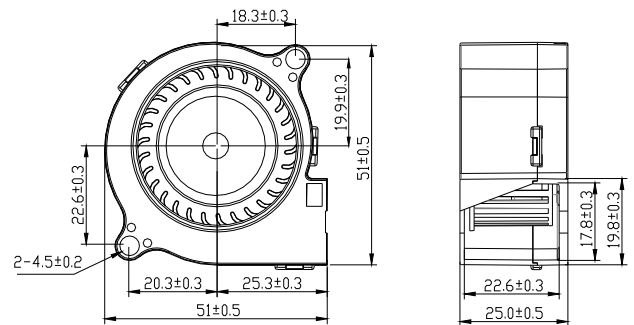
尺寸图 DIMENSIONS DRAWING
