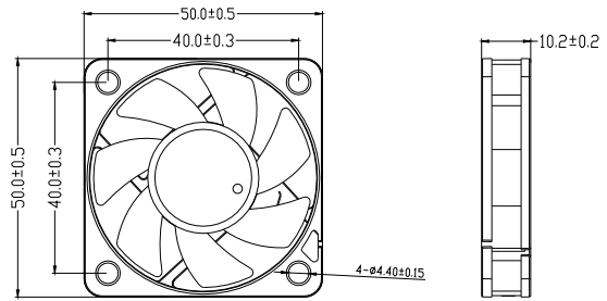
尺寸图 DIMENSIONS DRAWING
