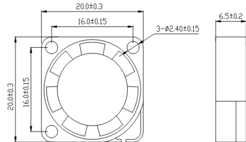
尺寸图 DIMENSIONS DRAWING
