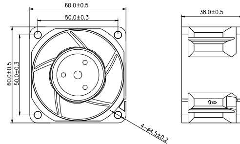
尺寸图 DIMENSIONS DRAWING
