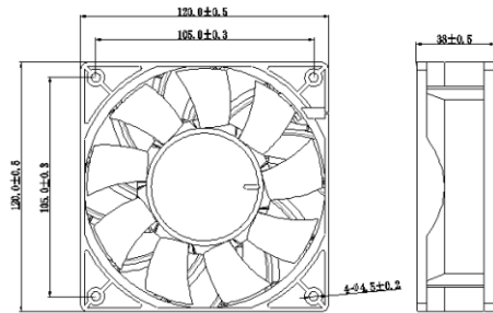
尺寸图 DIMENSIONS DRAWING
